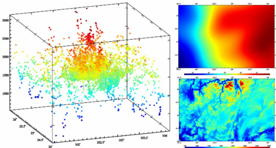
重力测点空间分布、模型大地水准面高m (右上) 和地面大地高m (右下)
