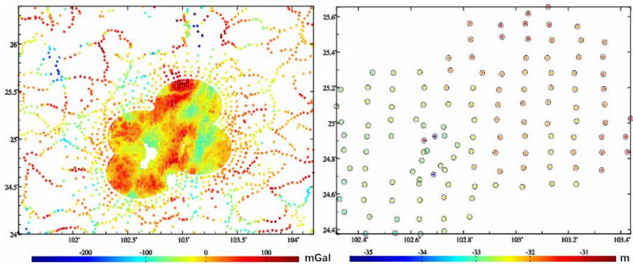
重力测点的实测扰动重力 (mGal) 与GNSS水准点的实测值 (m)
