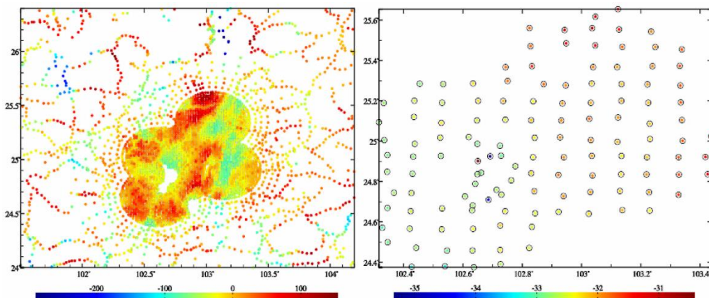
重力测点的实测扰动重力 (mGal) 与GNSS水准点的实测大地水准面高 (m)
