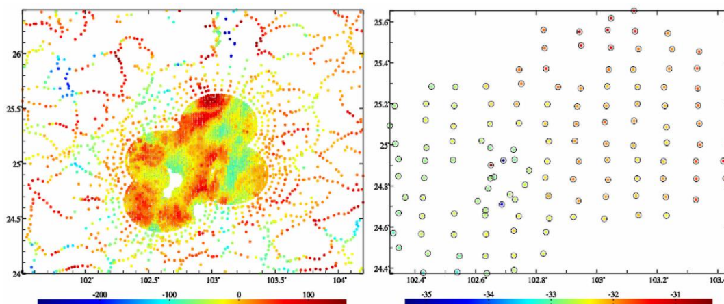
重力测点的实测扰动重力 (mGal) 与GNSS水准点的实测高程异常 (m)
