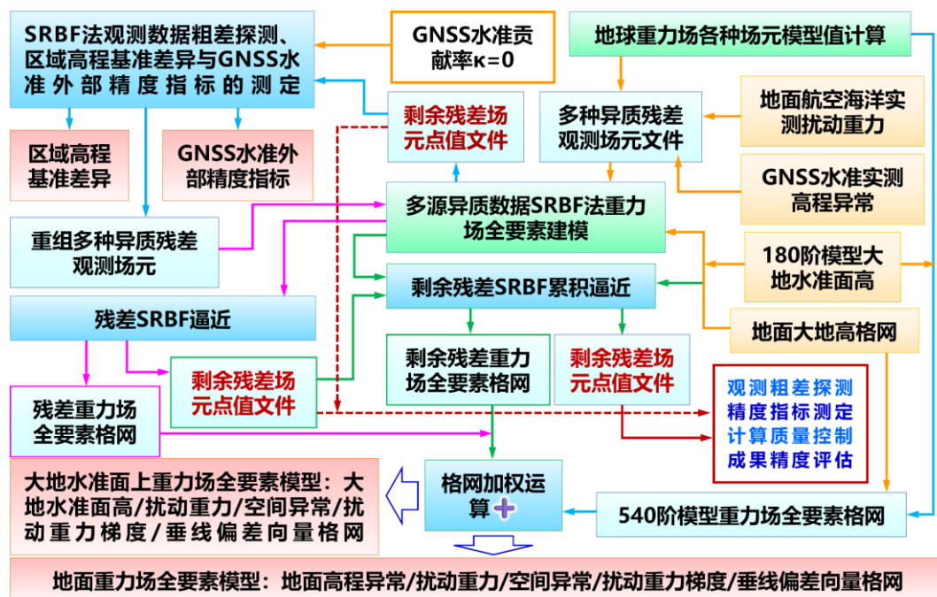
正常高系统谱域SRBF重力场全要素建模快捷流程
