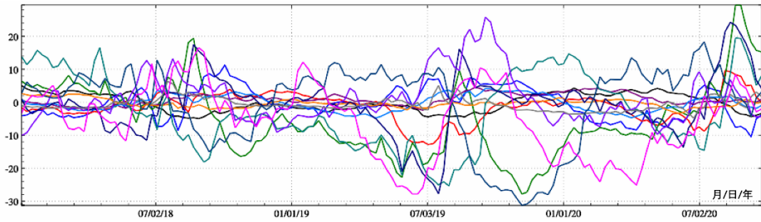
图 3.22 中国大陆陆地水变化负荷形变 (720 阶) -扰动重力梯度变化 10\mu\text{E}
