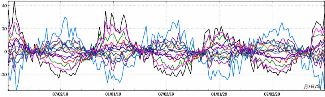
图 3.15 中国大陆地面大气压变化负荷形变 (180 阶) -扰动重力梯度变化 10\mu\text{E}
