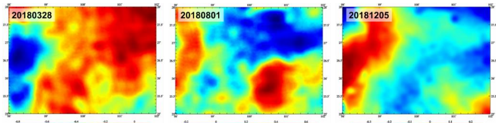
1'×1'地面大地高土壤水负荷效应(mm)残差格网时间序列
