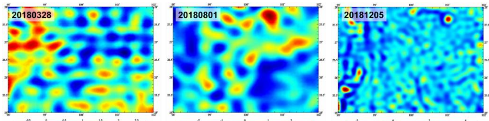
1'×1'重力梯度土壤水负荷效应(mE)残差格网时间序列
