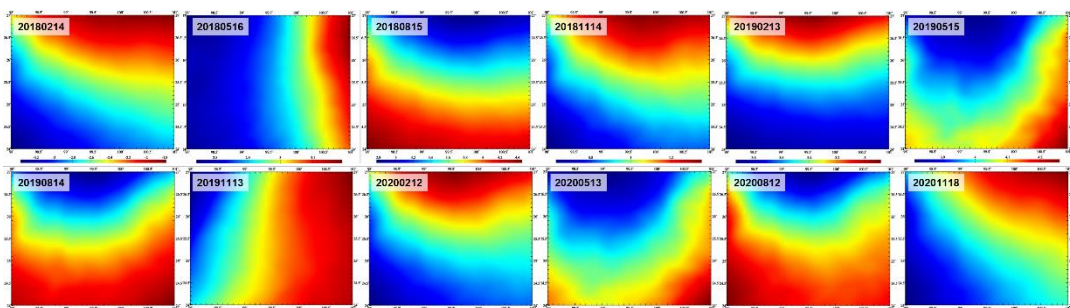
图 5.6 区域 3.75'x3.75'地面大地高大气压变化负荷效应 (mm) 格网时间序列
