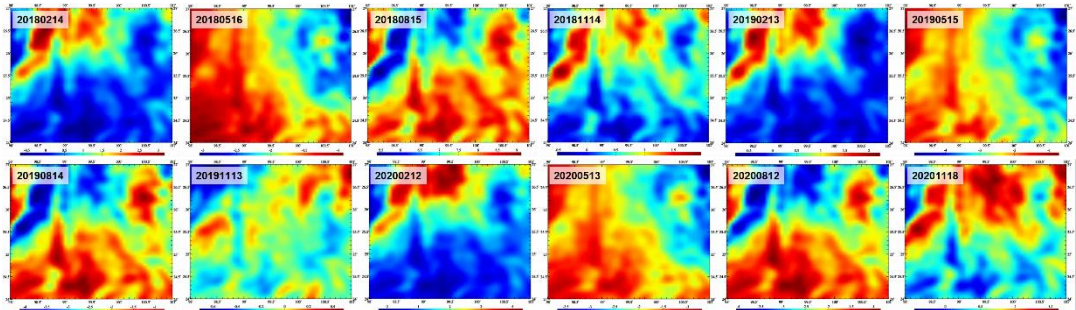
图 5.8 区域 3.75'x3.75'扰动重力梯度大气压变化负荷效应 (mE) 格网时间序列
