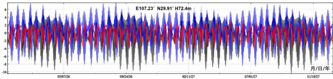
地面站点位移地球质心变化海潮负荷效应补偿预报值时间序列: 水平东 (mm), 水平北 (mm), 大地高 (mm)
