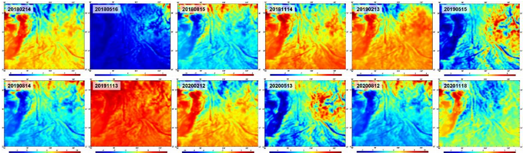
图 5.3 区域 3.75'\times 3.75' 地面大气压周变化 (hPa) 残差值格网时间序列
