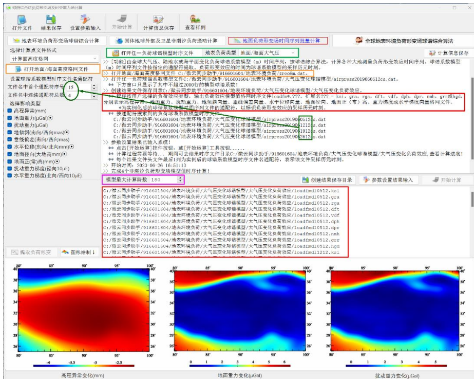
图 3.10 地面全要素大气压变化负荷效应格网时间序列计算
