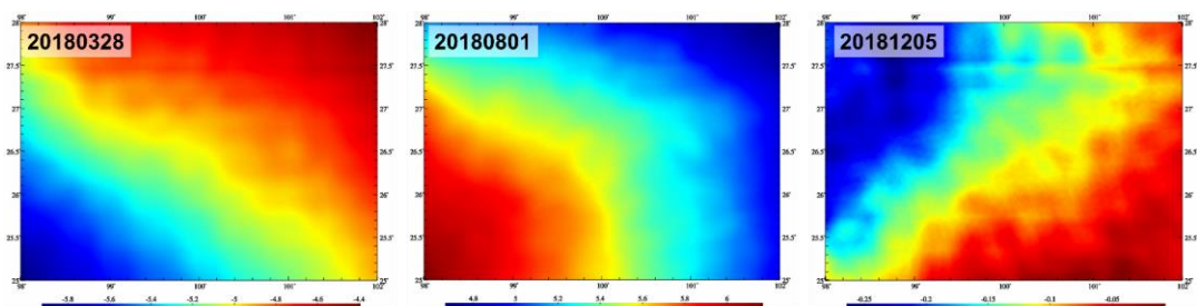
1'×1'大地水准面土壤水负荷效应(mm)格网时间序列成果
