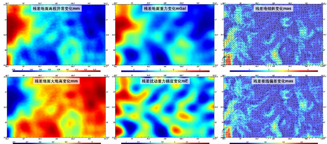
图 6.4 负荷 SRBF 谱域逼近的 30"×30"残差陆地水变化负荷形变场格网
