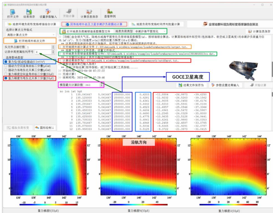
图 3.3 地球卫星海平面变化负荷摄动计算
