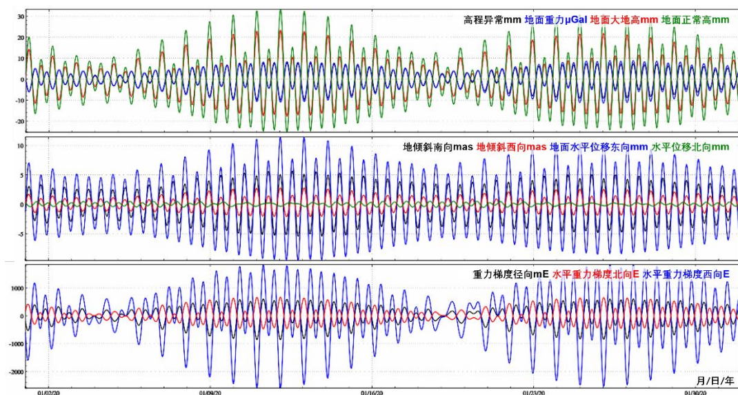
图 4.7 海岸 P_2 点大地测量全要素海潮负荷效应残差值时间序列
