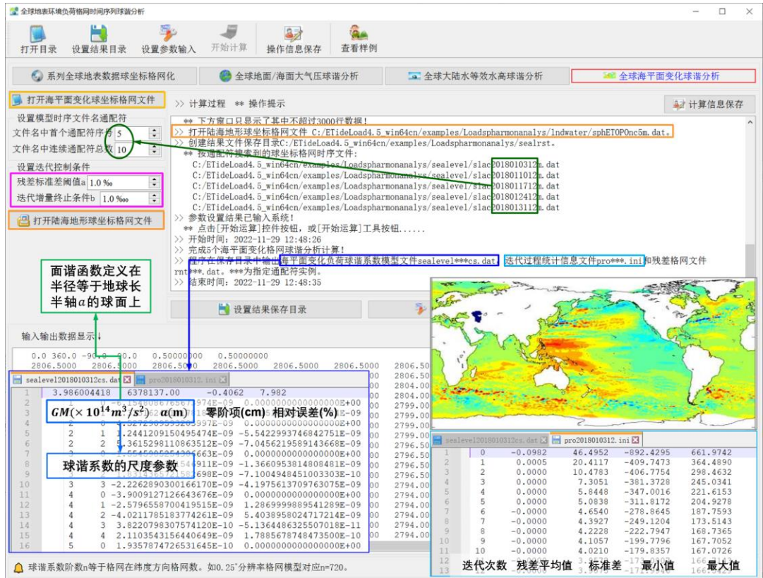
图 3.1 全球海平面变化球谐分析与负荷球谐模型构建
