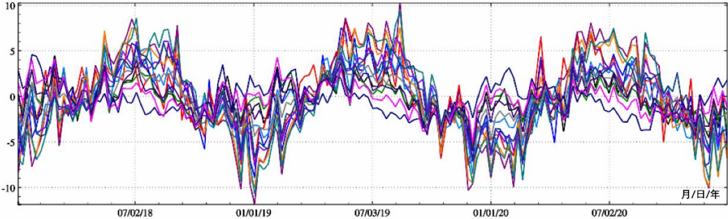
图 3.13 中国大陆地面大气压变化负荷形变 (180 阶) -地面重力变化 \mu\text{Gal}
