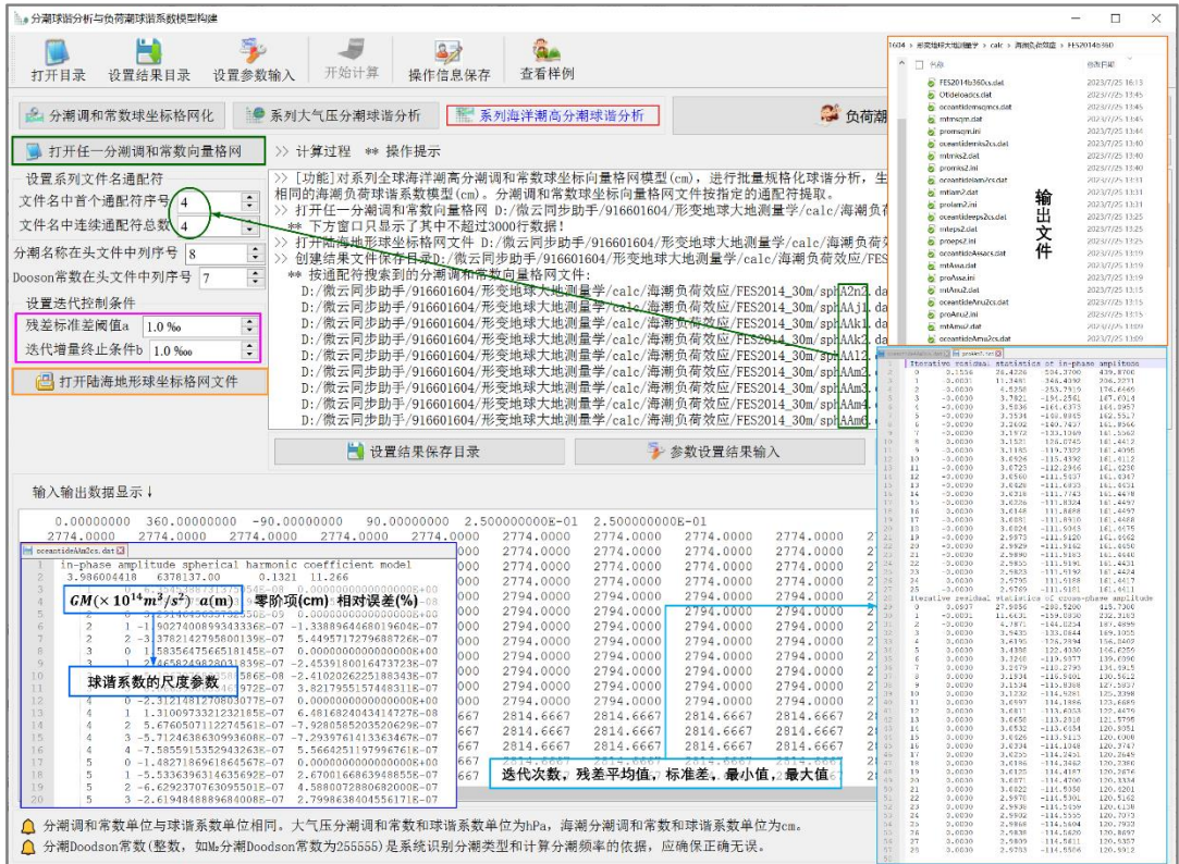
图 4.1 全球海潮调和与分析负负荷球谐系数模型构建程序
