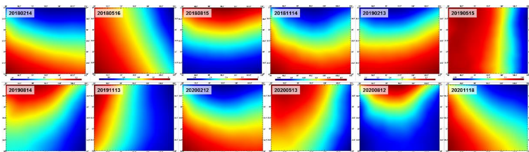
图 5.4 区域 3.75'x3.75'地面高程异常大气压变化负荷效应 (mm) 格网时间序列
