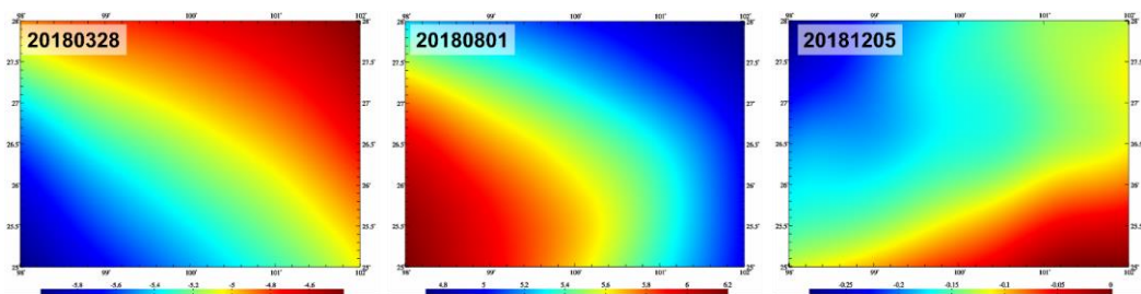
1'×1'大地水准面土壤水负荷效应参考模型值(mm)格网时间序列
