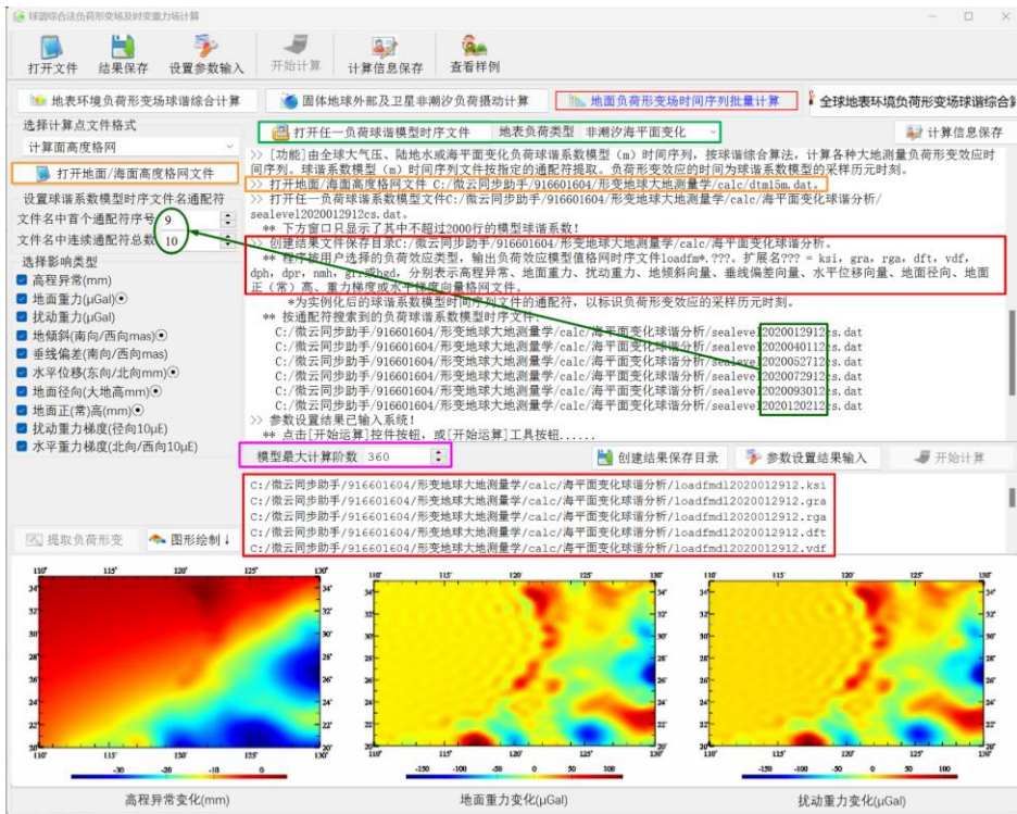
图 3.2 海平面变化负荷效应格网时间序列计算
