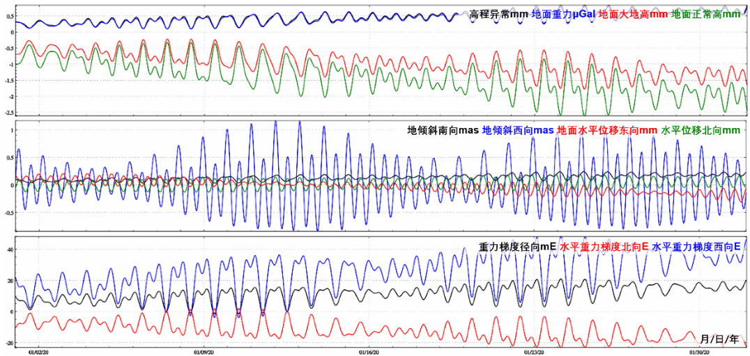
图 2 海岛 P_3 点大地测量全要素海潮负荷效应残差值时间序列
