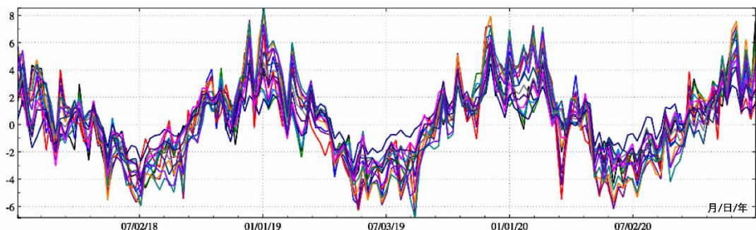
图 3.12 中国大陆地面大气压变化负荷形变 (180 阶) -大地水准面变化 mm
