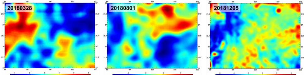
1'×1'地面重力土壤水负荷效应( \mu\text{Gal} )残差格网时间序列
