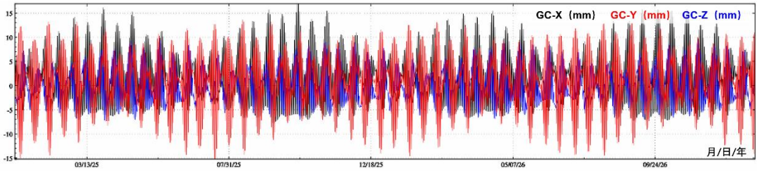
图 4.10 地球质心变化的海潮负荷效应时间序列预报
