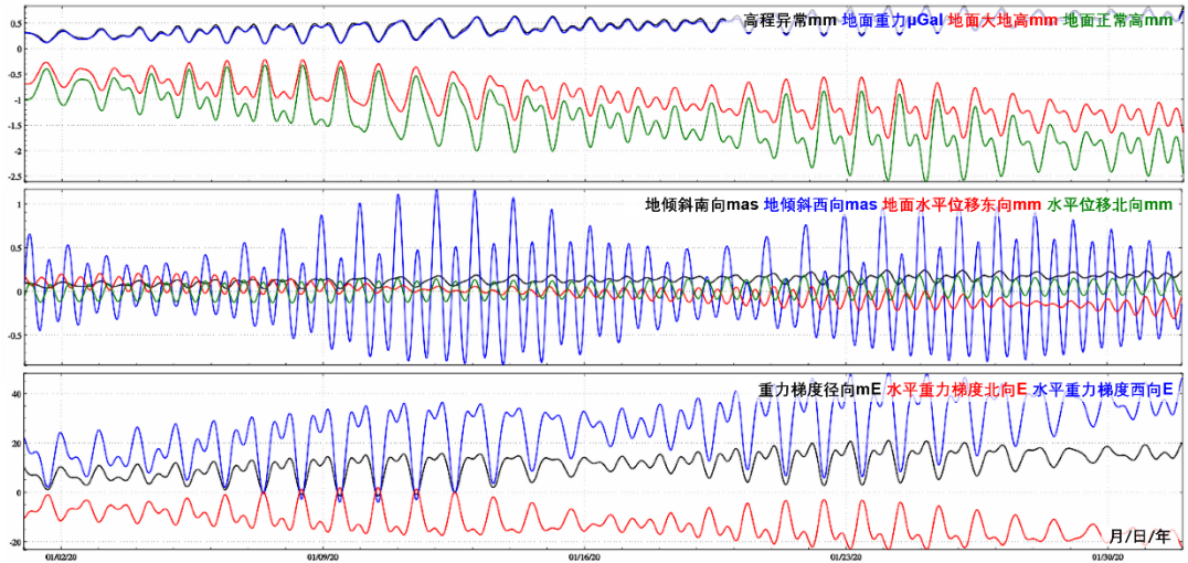
图 4.8 海岛 P_3 点大地测量全要素海潮负荷效应残差值时间序列
