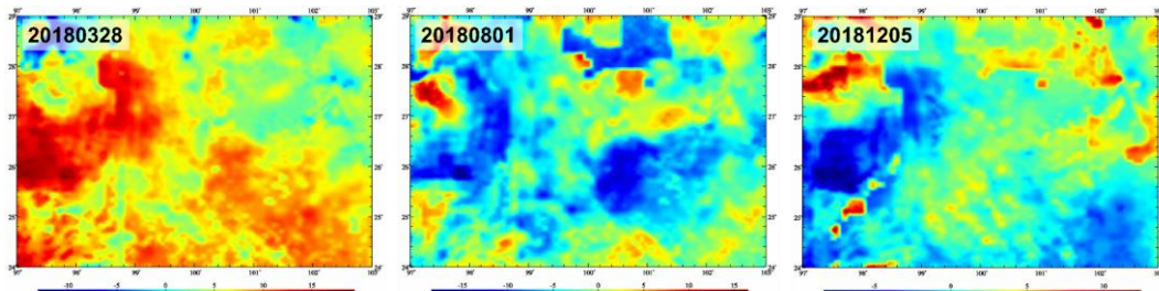
区域1'x1'土壤水等效水高(cm)残差格网时间序列
