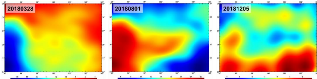
区域1'x1'土壤水等效水高(cm)参考模型值格网时间序列
