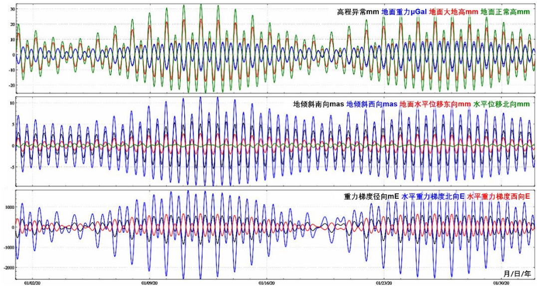
图 4.9 海岸 P_2 点各种大地测量海潮负荷效应精化值时间序列
