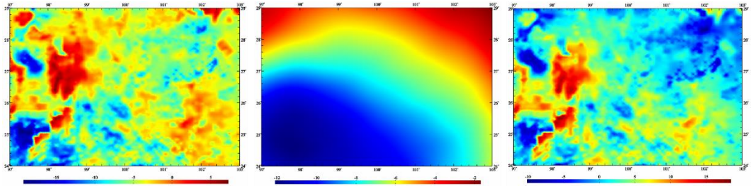
图 6.3 计算区域 1'×1'陆地水等效水高变化观测值、参考值与残差值 (cm) 格网
