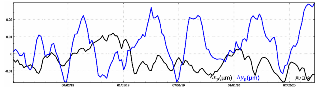
图 3.23 地球极移的陆地水变化负荷效应-相对于 2018 年平均位置
