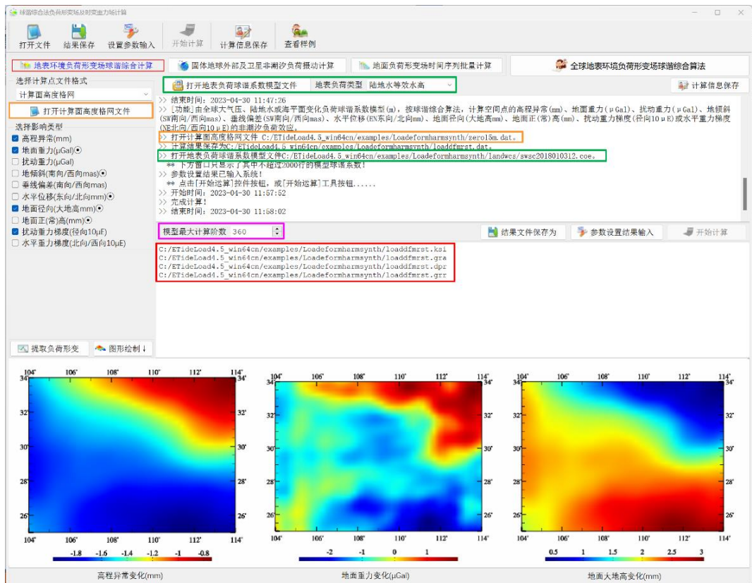
图 3.18 陆地水变化负荷效应球谐综合计算
