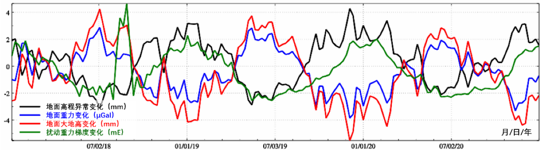
图 5.9 区域中心点处地面大地测量要素周变化大气压负荷效应时间序列
