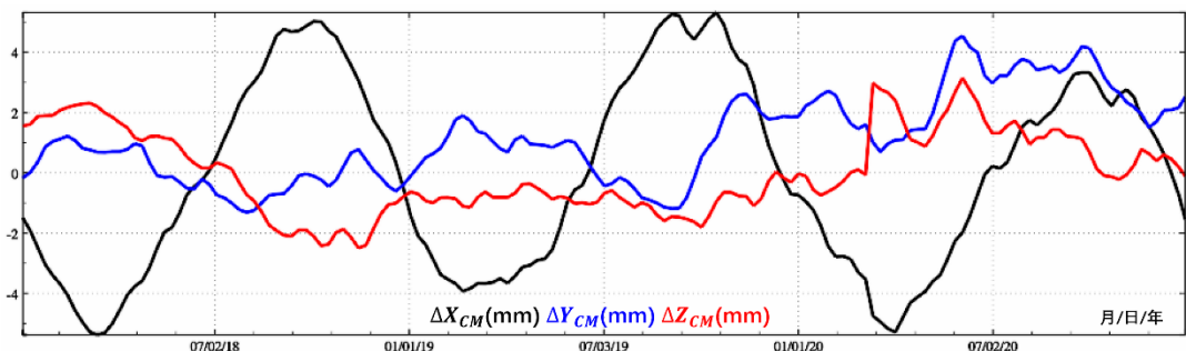
图 3.24 地球质心变化的海平面变化负荷效应-相对于 2018 年平均位置
