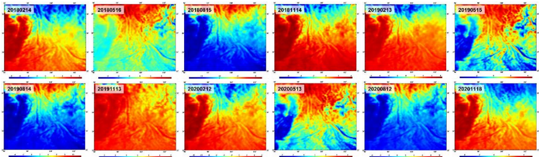
图 5.2 区域 3.75'\times 3.75' 地面大气压周变化 (hPa) 格网时间序列
