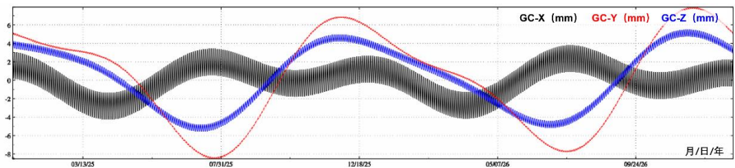
图 4.11 地球质心变化的大气压潮负荷效应时间序列预报
