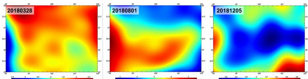
1'×1'地面重力土壤水负荷效应参考模型值 (μGal)格网时间序列
