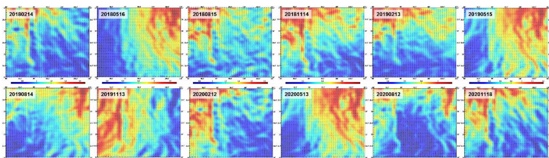
图 5.7 区域 3.75'x3.75'地倾斜大气压变化负荷效应 (mm) 格网时间序列
