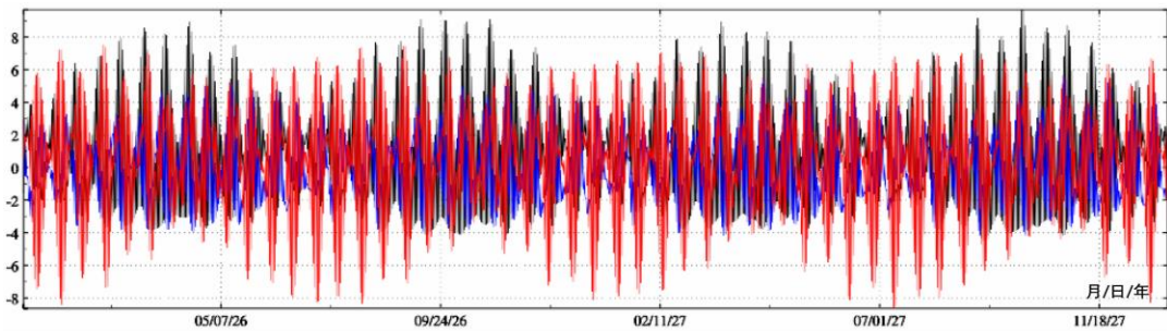
地球质心变化海潮负荷效应预报值时间序列 (mm): GC-X, GC-Y, GC-Z
