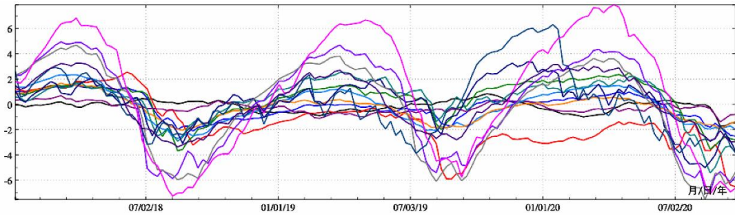
图 3.21 中国大陆陆地水变化负荷形变 (720 阶) -地面大地高变化 mm
