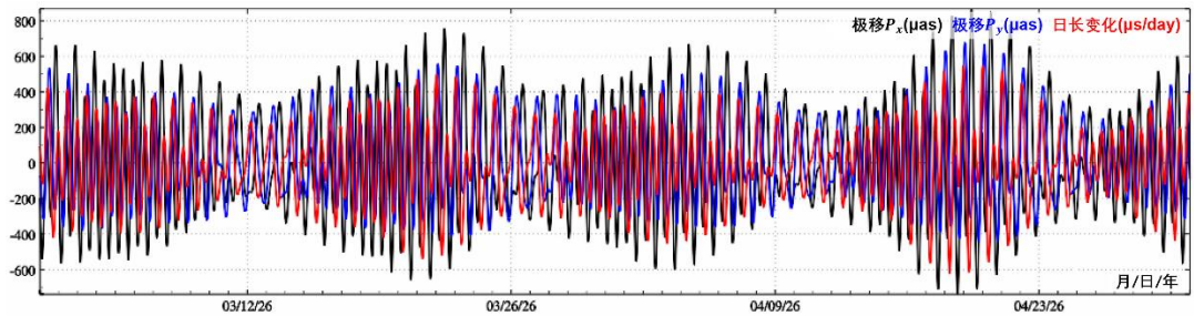
图 2.4 地球自转参数的周日/半日潮汐效应预报时间序列
