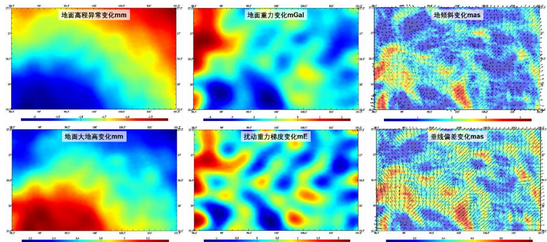
图 6.5 移去-负荷 SRBF 谱域逼近-恢复法计算的 30"×30"陆地水变化负荷形变场格网
